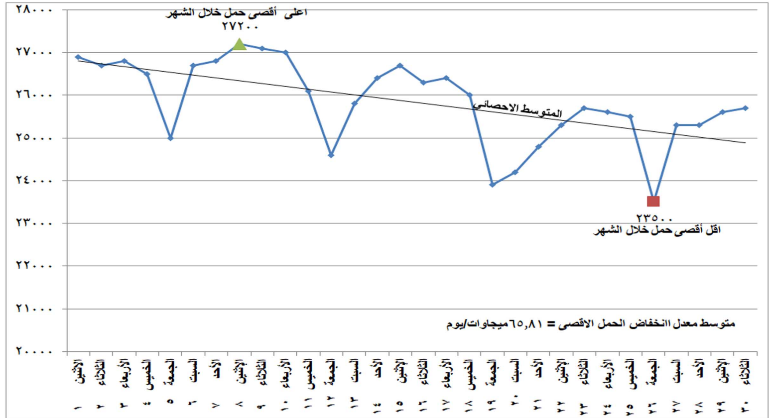
شكل (١) تطور الحمل الاقصى اليومي خلال شهر نوفمبر ٢٠٢١
