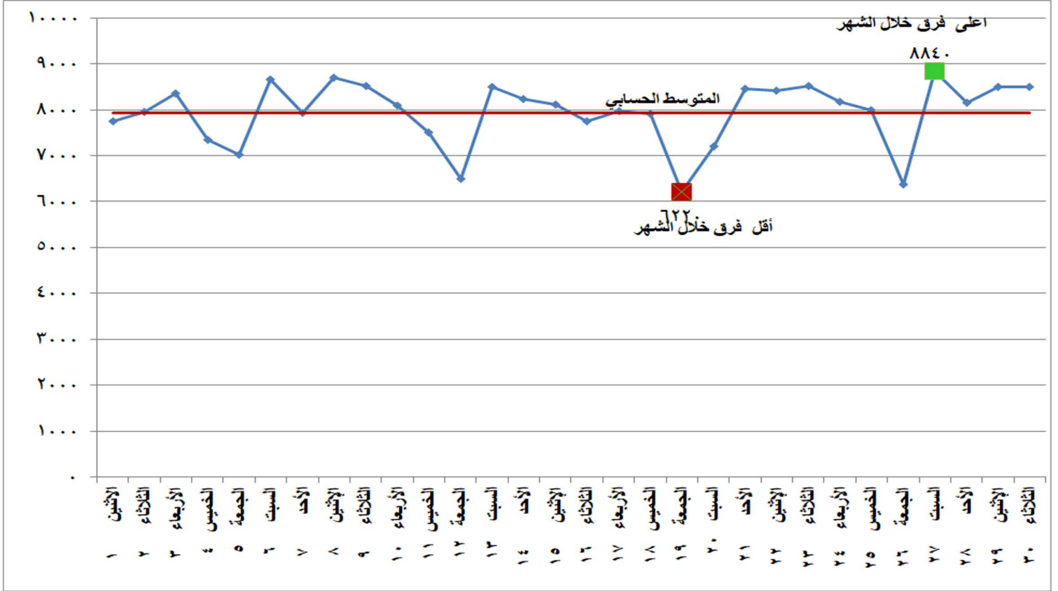
شكل (٣) الفرق بين أقصى وأدنى حمل خلال شهر نوفمبر ٢٠٢١
