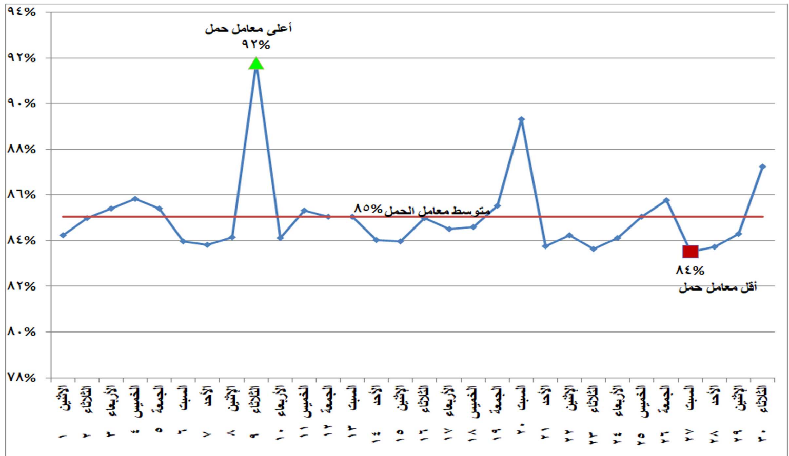
شكل (١٢) إجمالي معامل الحمل لوحدات الانتاج خلال شهر نوفمبر ٢٠٢١
