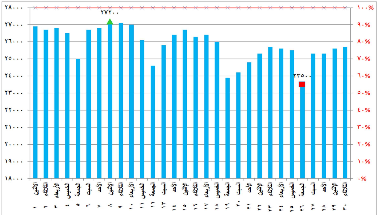
شكل (٥) قدرات الانتاج المتاحة ونسبتها للحمل الأقصى خلال شهر نوفمبر ٢٠٢١
