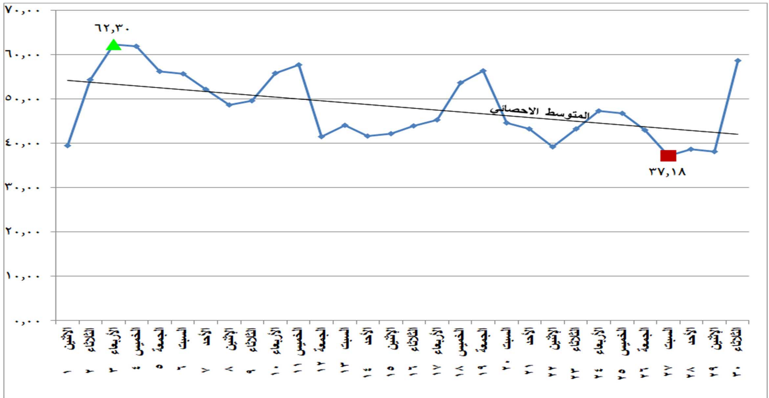
شكل (٢١) الطاقة الكهربائية المنتجة من المصادر غير الحرارية خلال شهر نوفمبر ٢٠٢١
