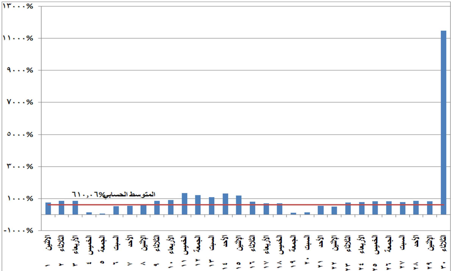
شكل (٢٠) نسب التغير في استخدام المازوت في إنتاج الطاقة الكهربائية خلال شهر نوفمبر ٢٠٢١ مقارنة بالشهر المماثل من العام السابق
