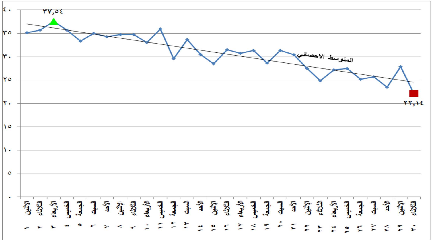
شكل (٢٣) الطاقة الكهربائية المنتجة من المصادر المائية خلال شهر نوفمبر ٢٠٢١
