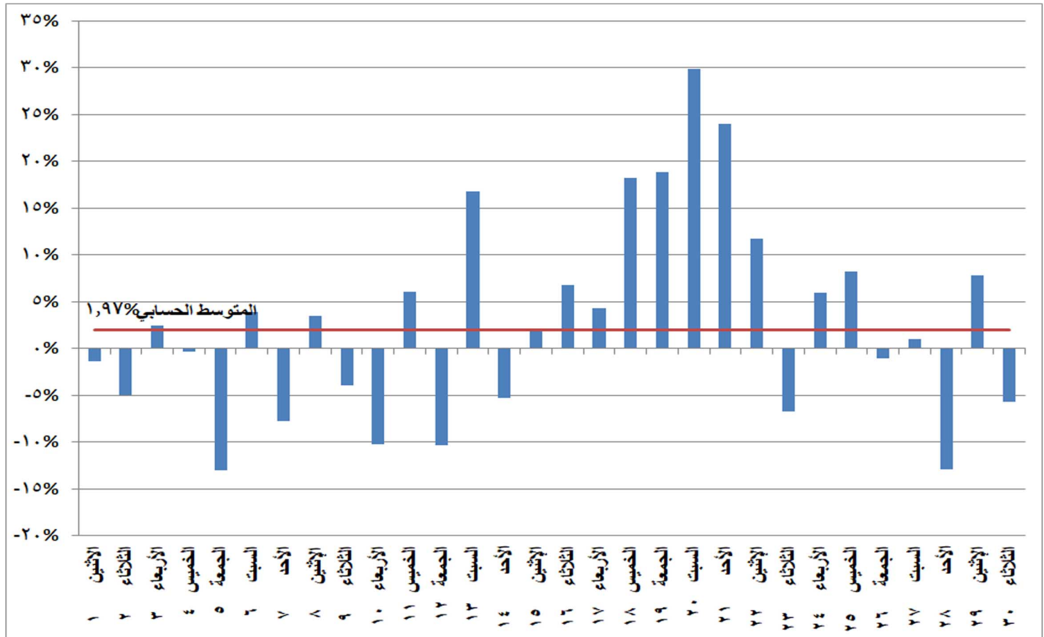
شكل (٢٤) نسب التغير في استخدام المصادر المائية في إنتاج الطاقة الكهربائية خلال شهر نوفمبر ٢٠٢١ مقارنة بالشهر المماثل من العام السابق
