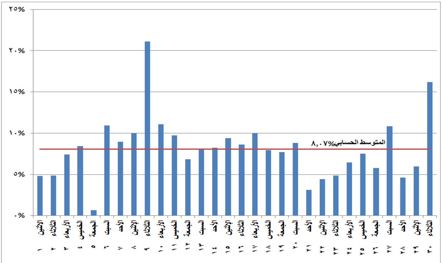
شكل (١٦) نسب التغير في الطاقة الكهربائية المنتجة خلال شهر نوفمبر ٢٠٢١ مقارنة بالشهر المماثل من العام السابق
