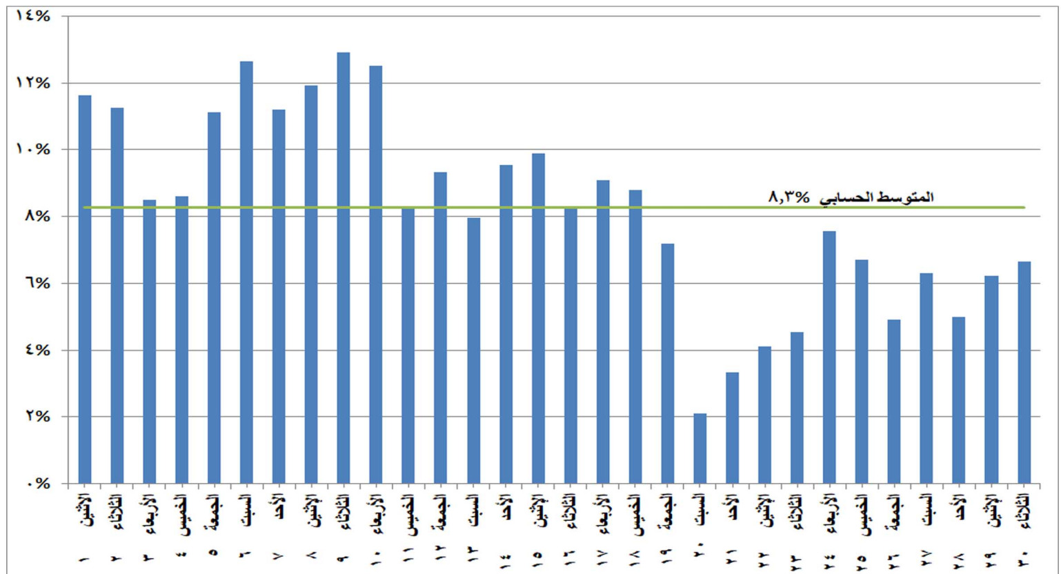
شكل (٩) النسب المئوية للتغير في الحمل الاقصى خلال شهر نوفمبر ٢٠٢١ مقارنة باليوم المماثل من العام الماضي
