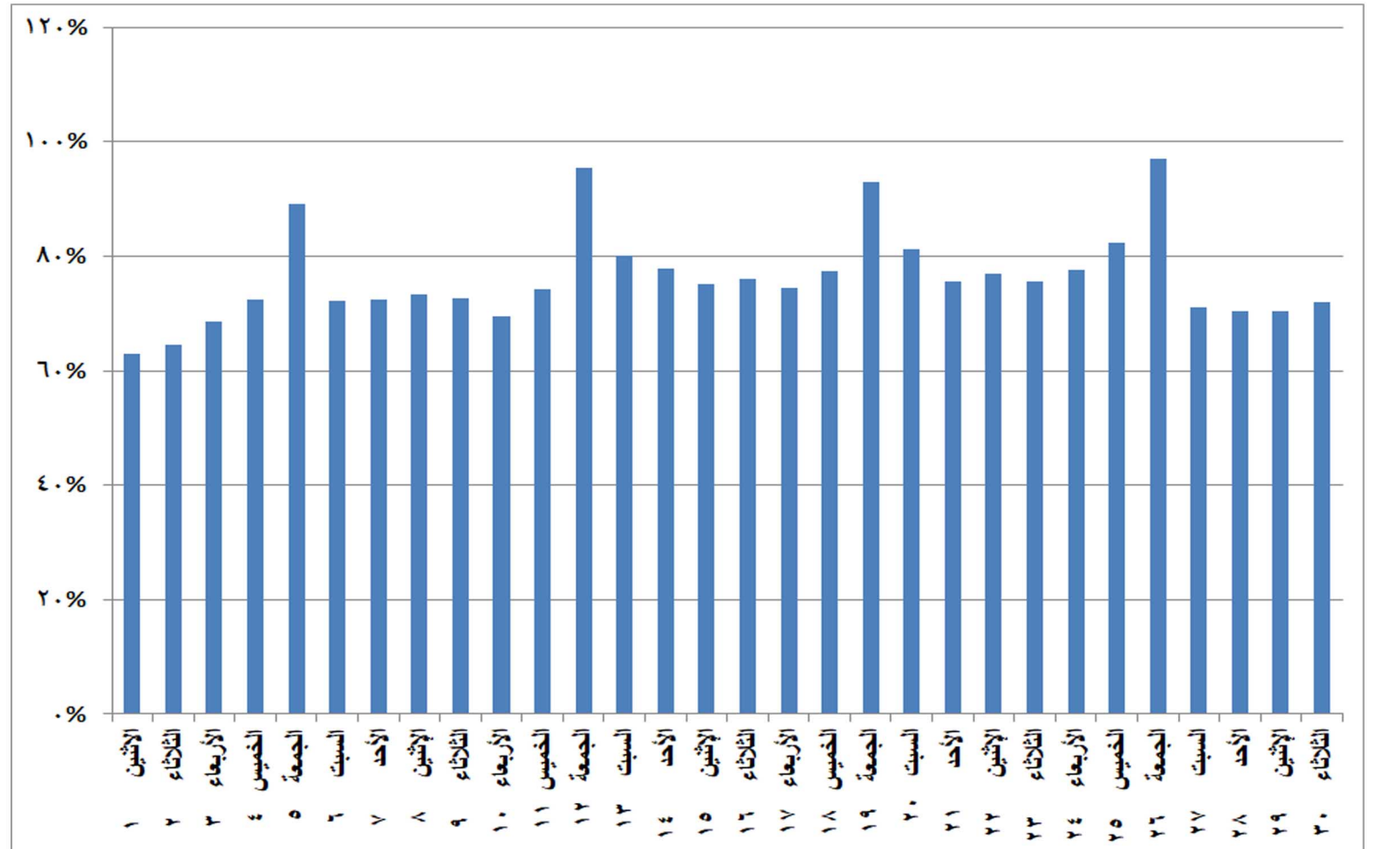
شكل (٢٨) نسب الفائض للحمل الاقصى المسجل يوميا خلال شهر نوفمبر ٢٠٢١
