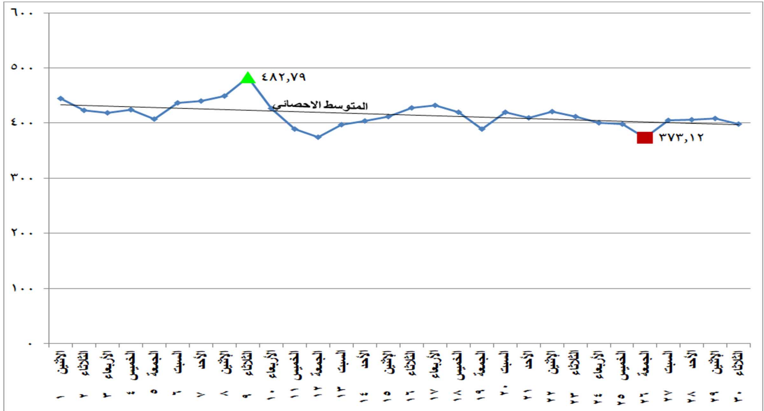
شكل (١٧) الطاقة الكهربائية المنتجة من الغاز الطبيعي خلال شهر نوفمبر ٢٠٢١
