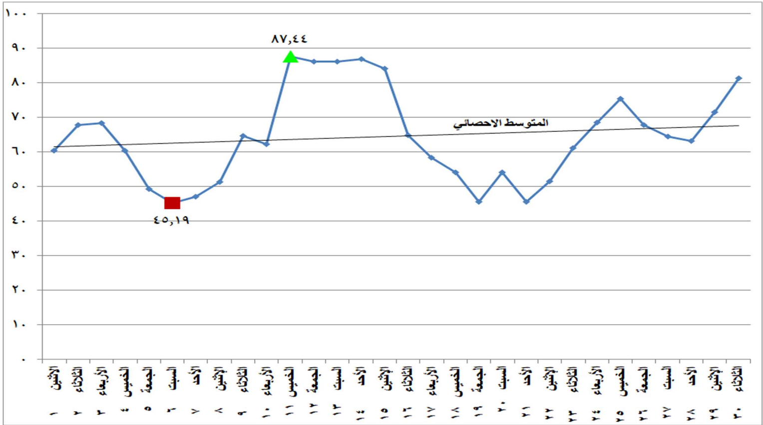
شكل (١٩) الطاقة الكهربائية المنتجة من المازوت خلال شهر نوفمبر ٢٠٢١
