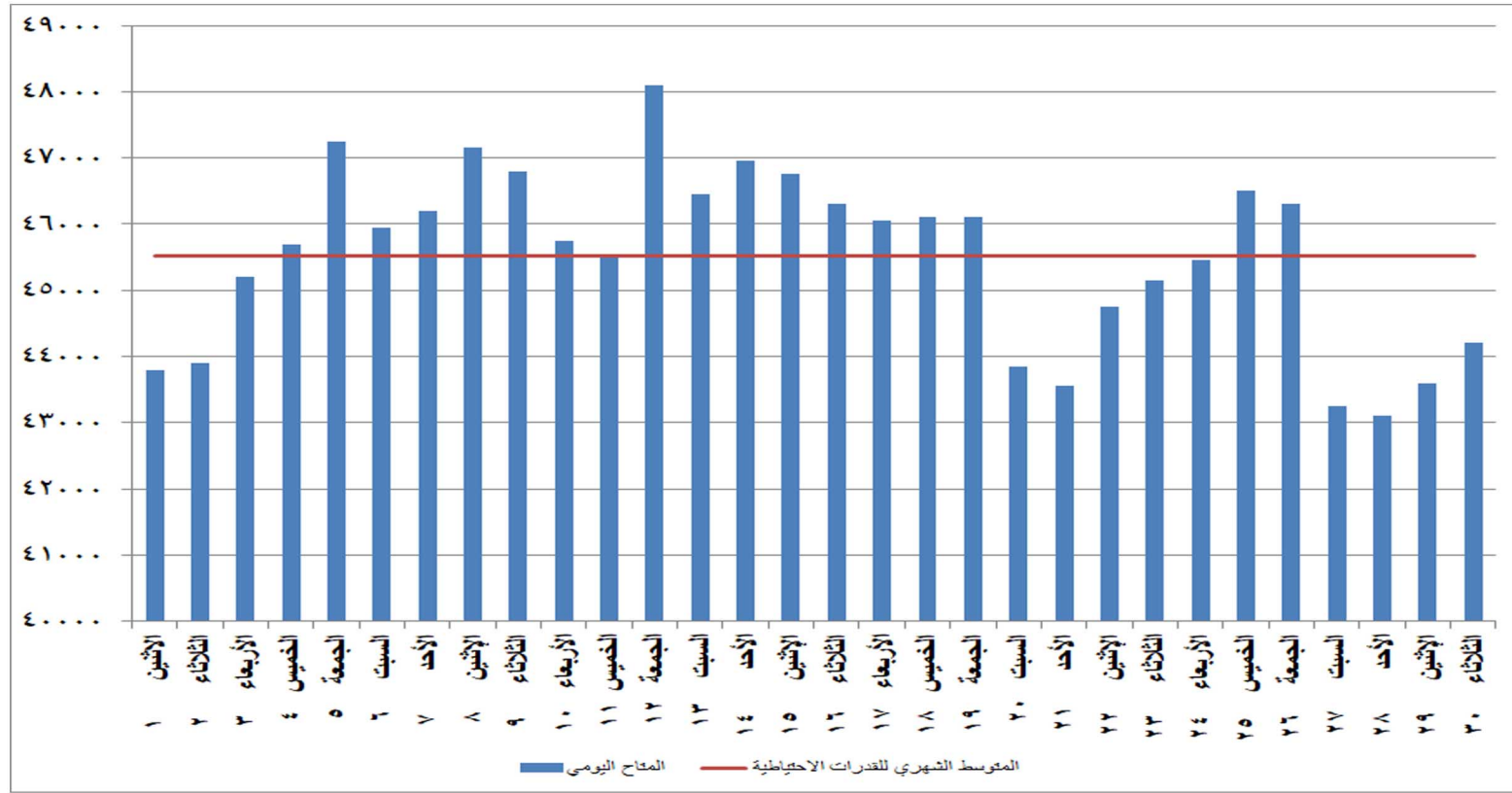
شكل (٢٧) القدرات المتاحة يوميا والمتوسط الشهري للقدرة الاحتياطية خلال شهر نوفمبر ٢٠٢١
