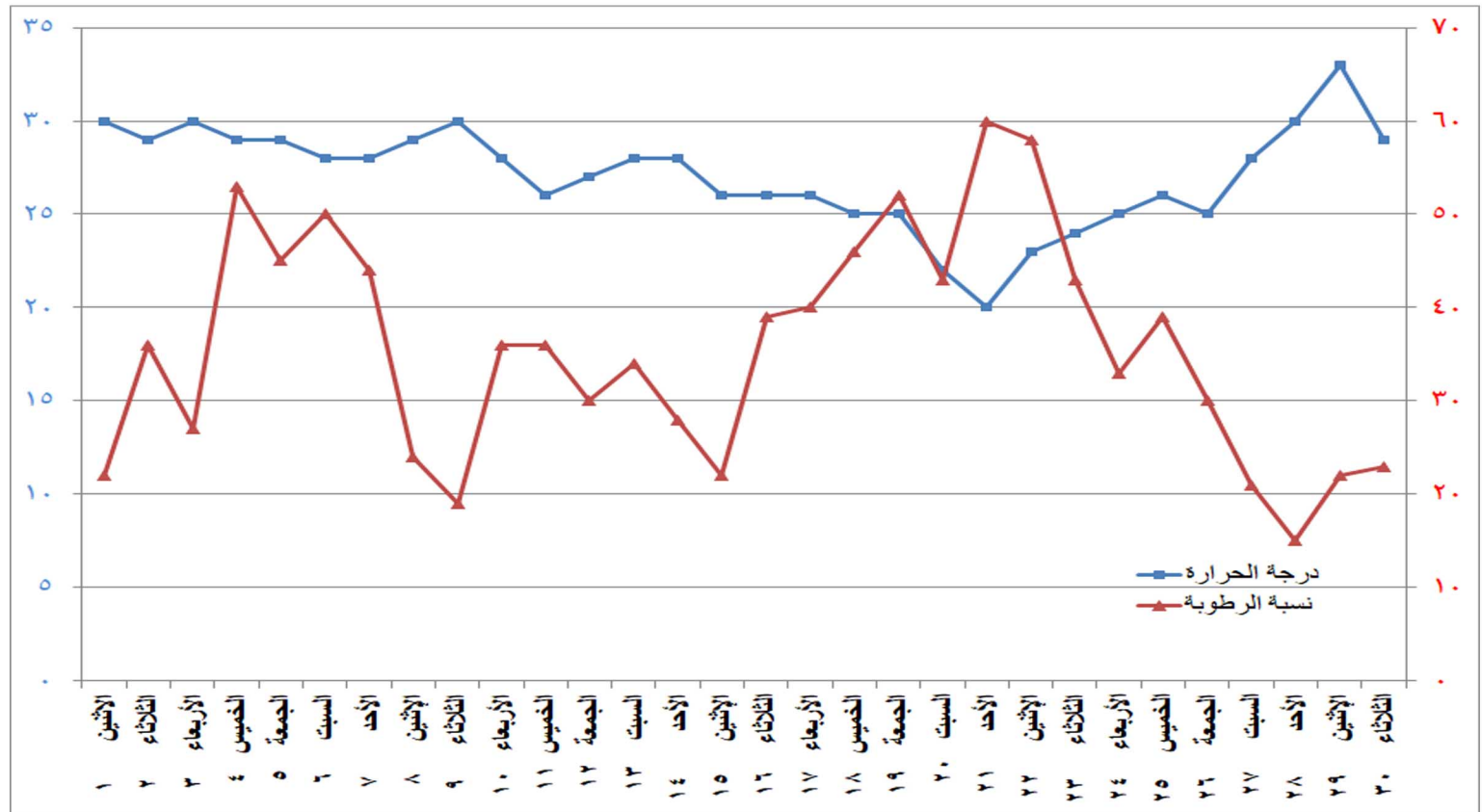
شكل (١١) التغيير في درجة الحرارة والرطوبة النسبية خلال شهر نوفمبر ٢٠٢١
