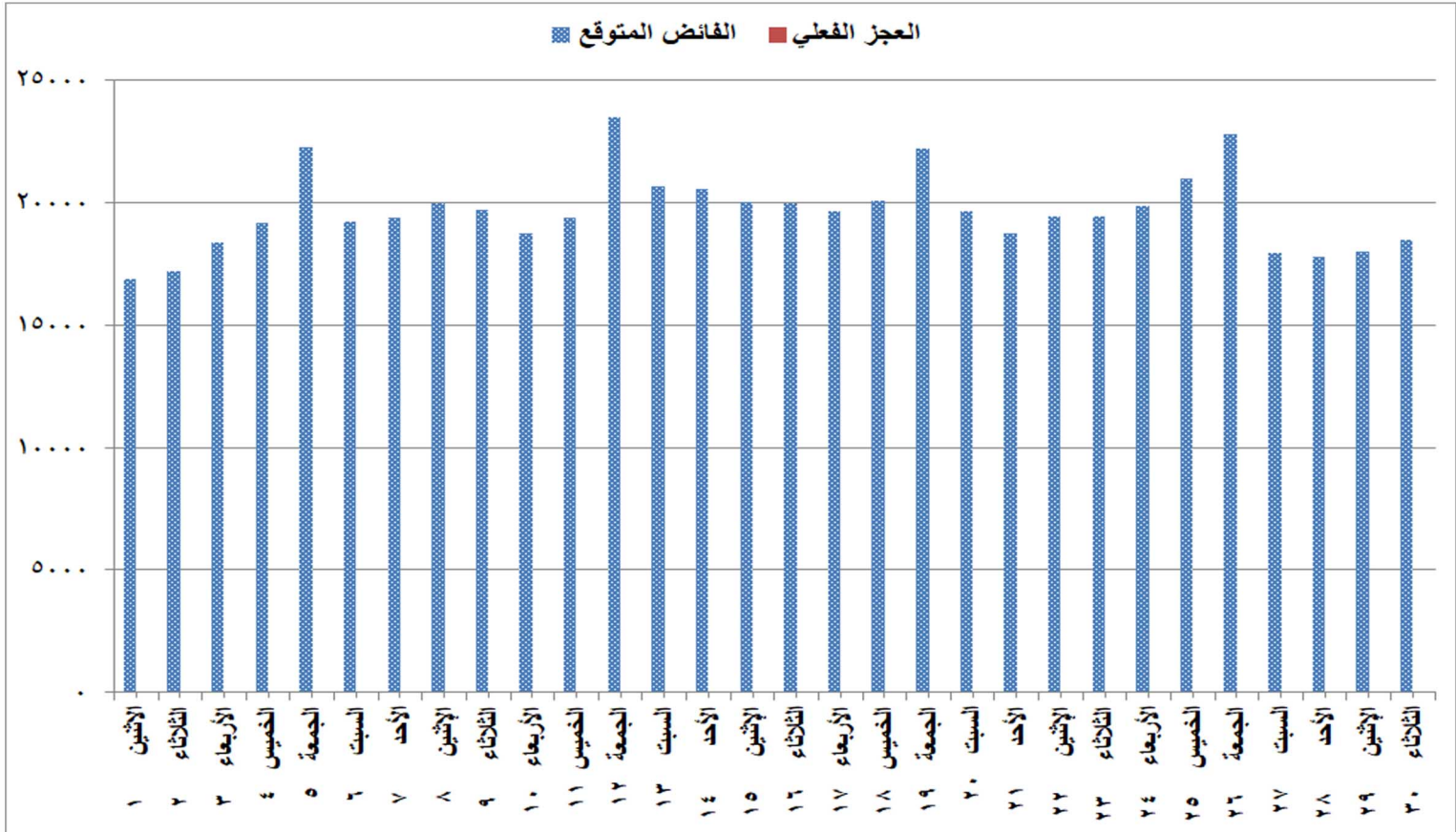
شكل (٧) الفائض والعجز المتوقع للقدرات خلال شهر نوفمبر ٢٠٢١
