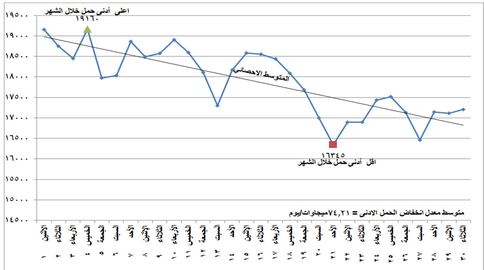
شكل (٢) تطور الحمل الادنى اليومي خلال شهر نوفمبر ٢٠٢١
