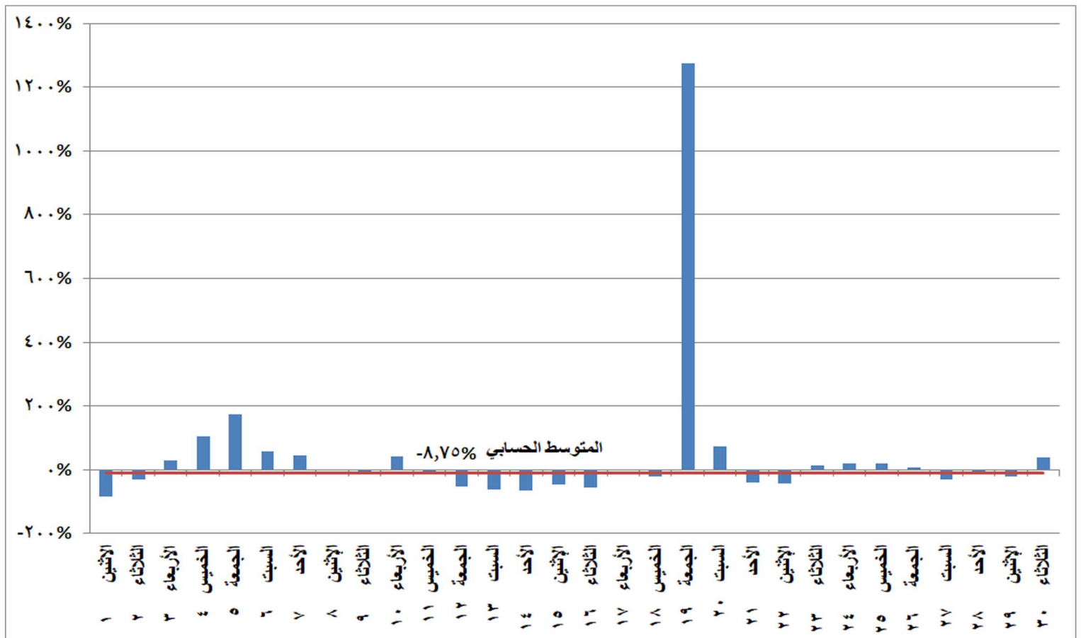
شكل (٢٦) نسب التغير في استخدام الرياح والشمس في إنتاج الطاقة الكهربائية خلال شهر نوفمبر ٢٠٢١ مقارنة بالشهر المماثل من العام السابق
