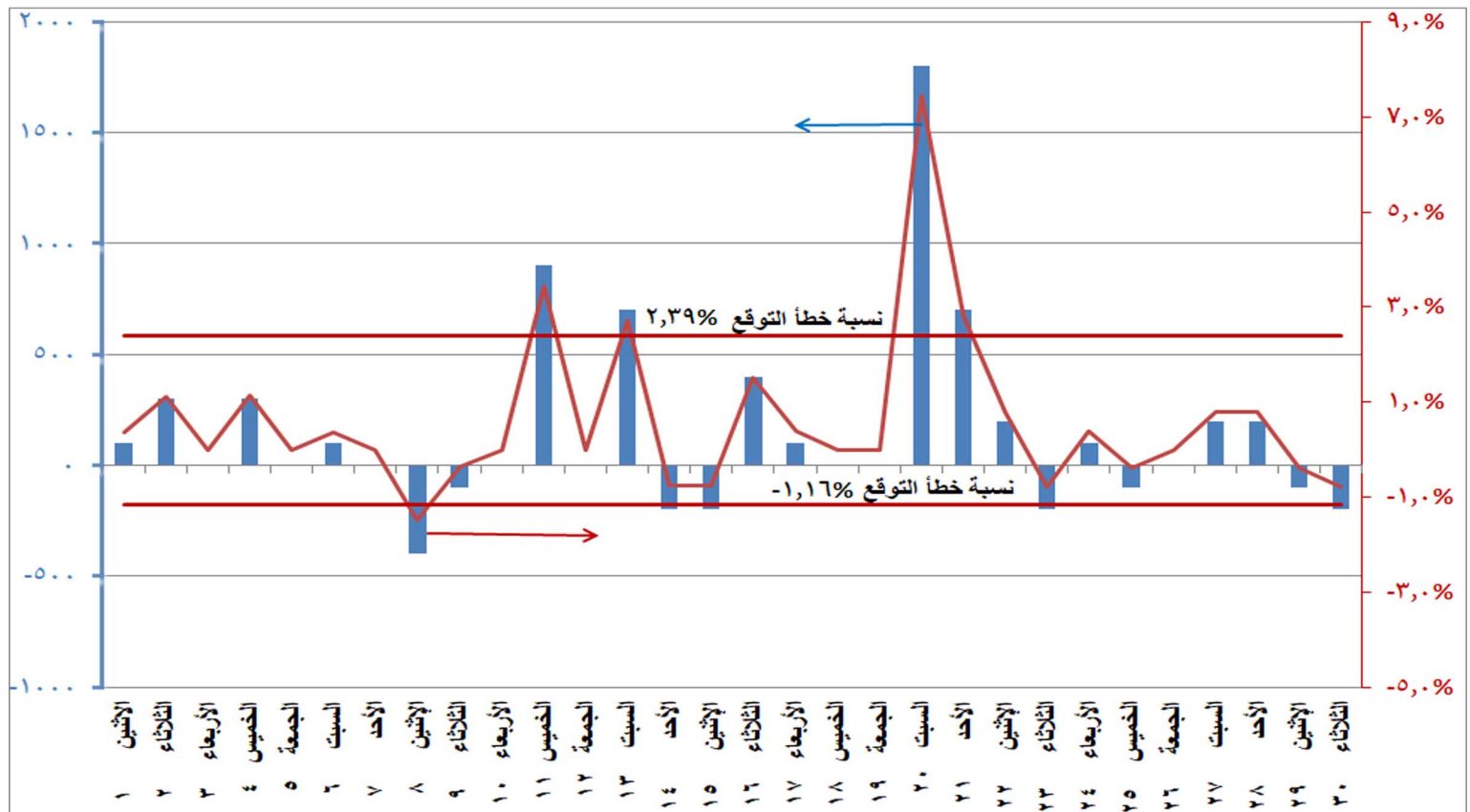
شكل (١٠) الفرق بين الحمل الأقصى المتوقع والمسجل فعليا ونسبة الفرق إلى الحمل المسجل فعليا خلال شهر نوفمبر ٢٠٢١
